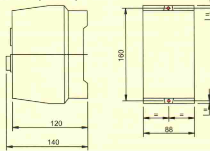
KD-1L. (25/32)
