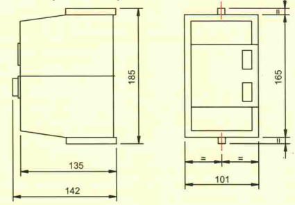
KD-1L. (9/12/18)
