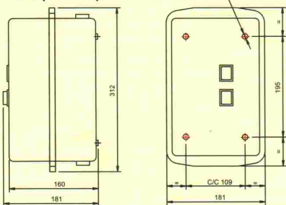
KD-1L. (40 / 95)
